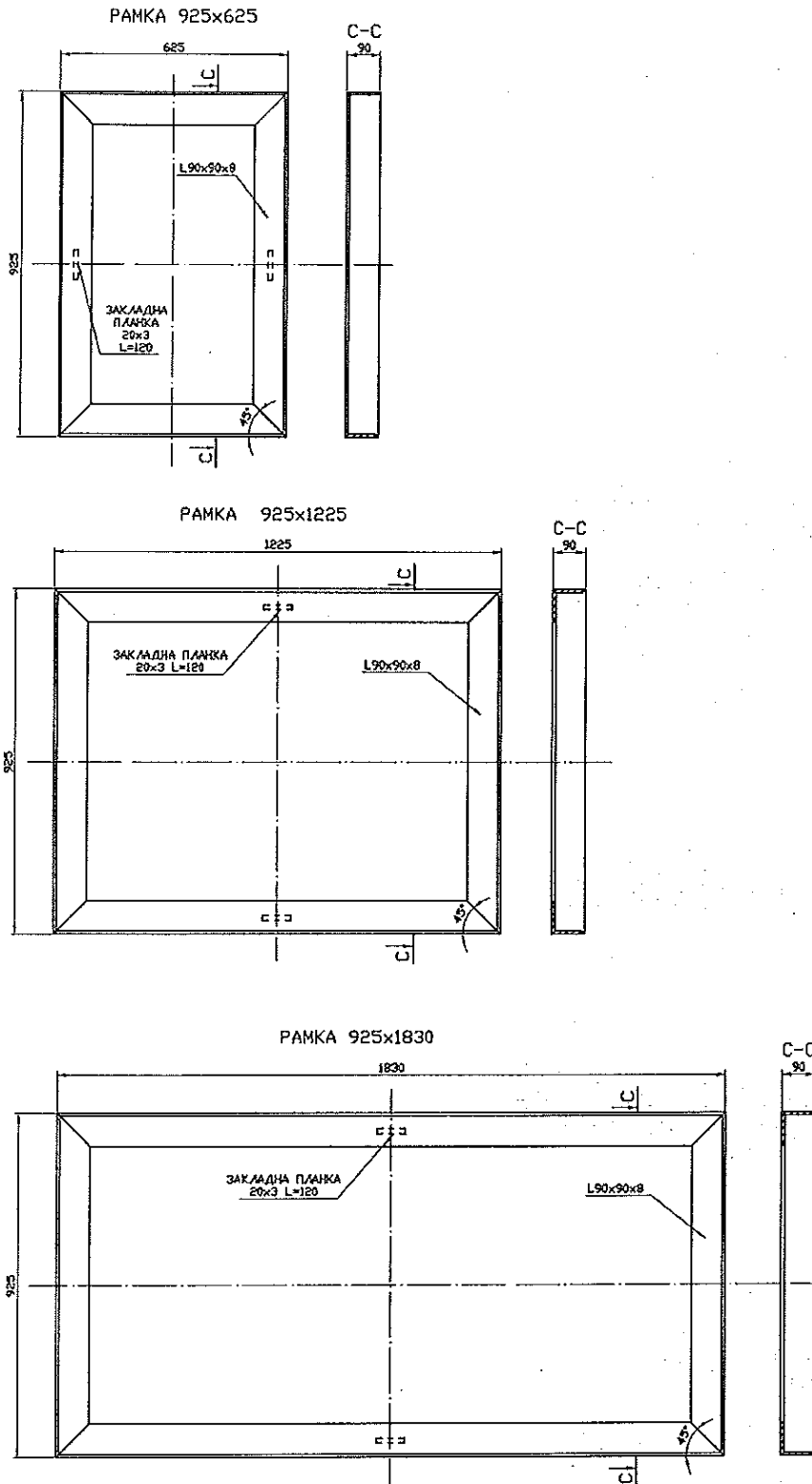
Фиг. 1 – Размери на метални рамки за капаци за кабелни шахти
